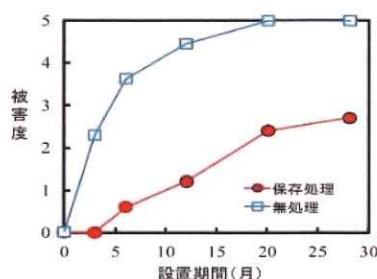
図 腐朽促進試験における被害度の経時変化 (カラマツ辺材) 2)
